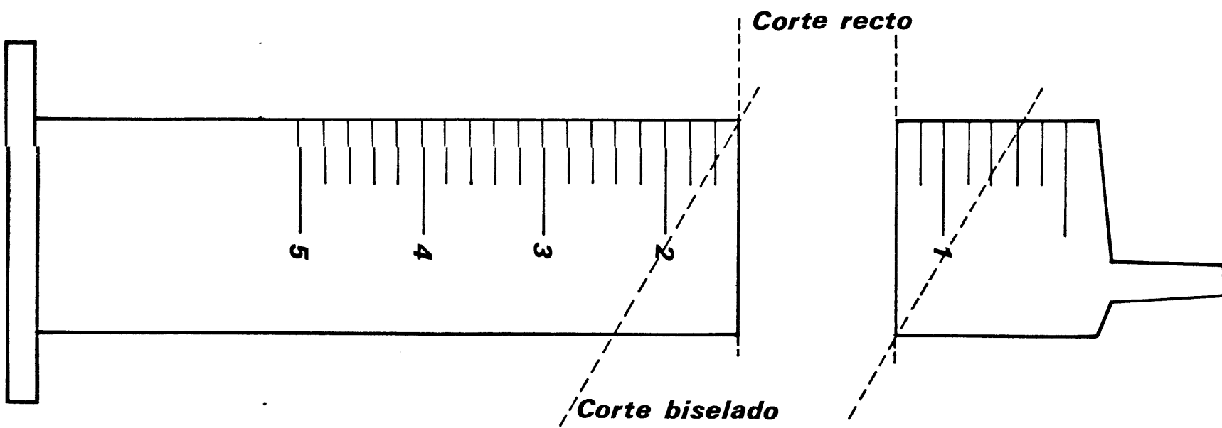
Cuerpo de jeringuilla, suprimido el fondo (Puede emplearse como cánula provisional)
